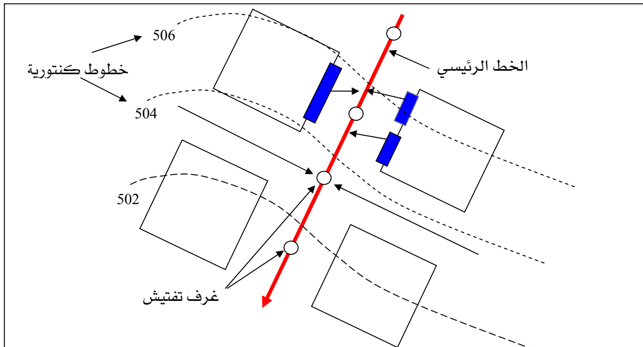
شكل (٤.١): خريطة كنتورية تبين تخطيط الشبكة
